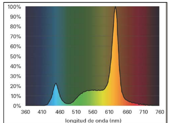
Figura 13. Espectro total LED con énfasis en es espectro
