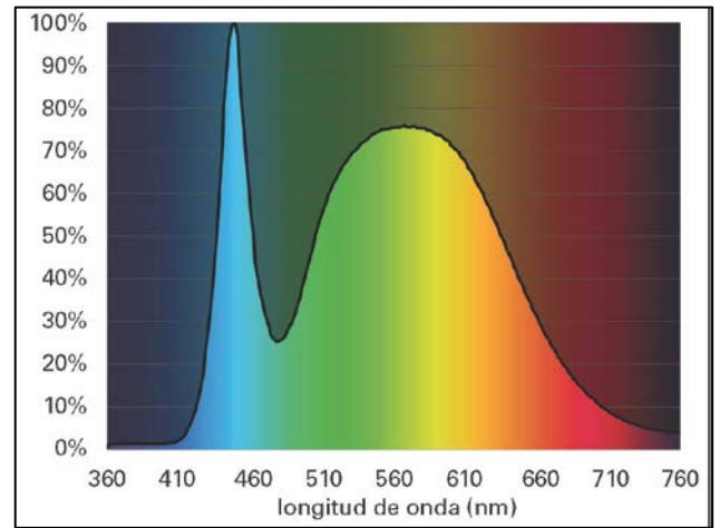
Figura 11. Espectro frío (5000K) luz LED.
