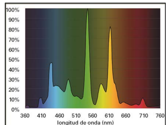
Figura 10. Espectro frío (5000K) luz fluorescente.
