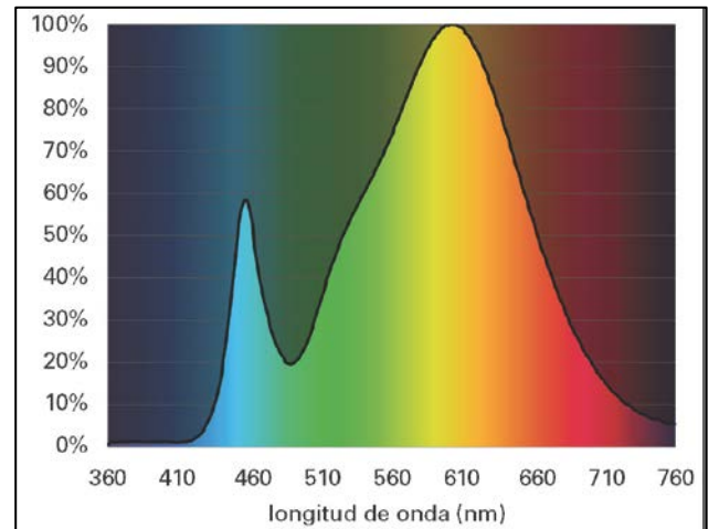
Figura 12. Espectro cálido (2700K) luz LED.
