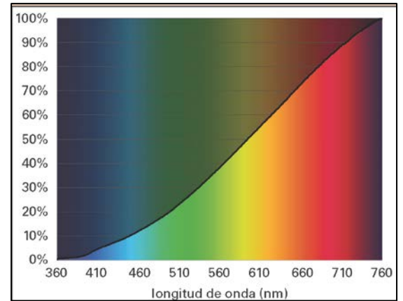
Figura 8. Espectro de la luz incandescente.
