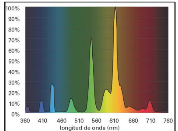
Figura 9. Espectro cálido (2700K) luz fluorescente.
