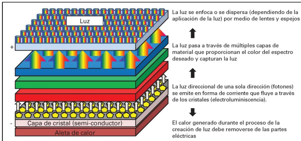
Figura 17. Como se crea la luz LED.
